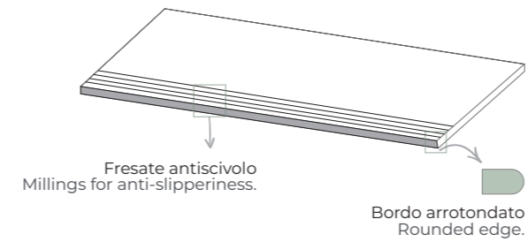
BORDO ANTISCIVOLO ANTI-SKID EDGE
